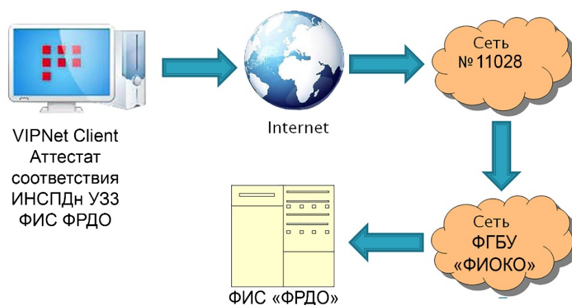
Рисунок 2 – Схема подключения к ФИС ФРДО
